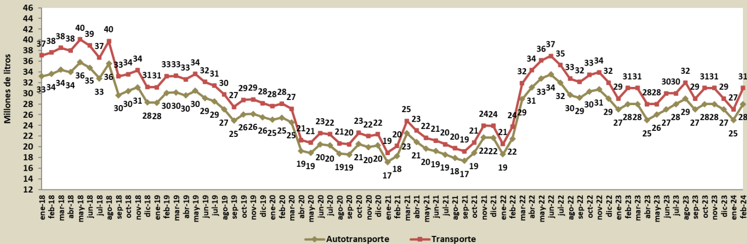
Consumo de Diesel (millones de litros diarios) 2018-2024
